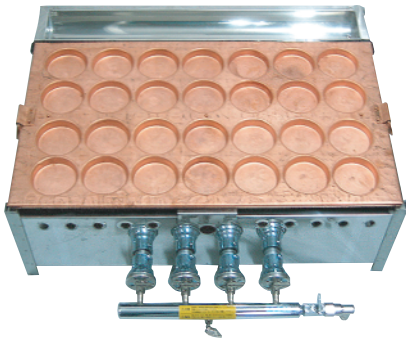
できあがり個数14個の回転焼き台 [28穴(7穴×4行)]
